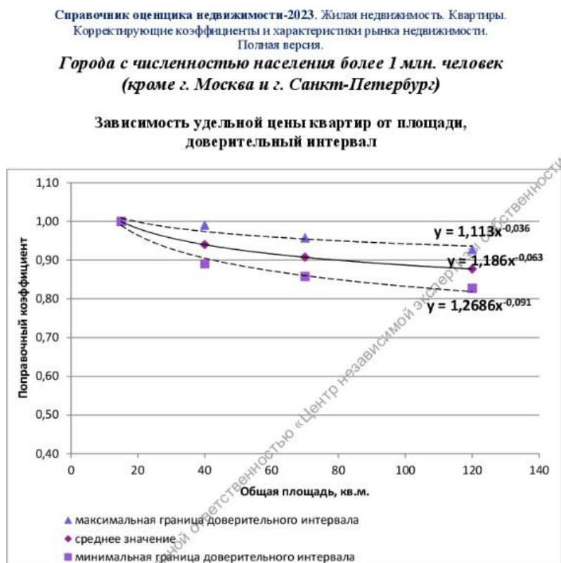
Рис. 61. Зависимость удельной цены квартир от площади, данные по городам с численностью населения более 1 млн. человек (кроме г. Москва и г. Санкт-Петербурга). Доверительный интервал 53 .
